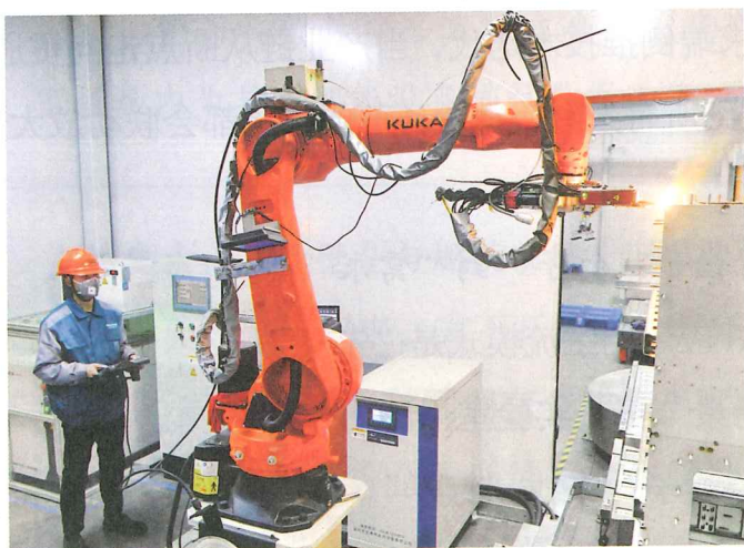
2025年3月6日，在四川成都双流经济开发区的特锐德川开电气有限公司生产车间内，气箱机器人正在进行焊接作业。 李向雨/摄
