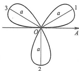
(16) 三叶玫瑰线
