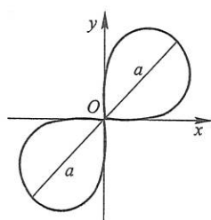
(13) 伯努利双纽线
