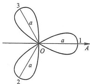
(15) 三叶玫瑰线
