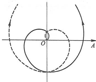
(10) 阿基米德螺线
