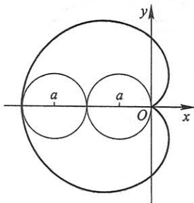
(9) 心形线(外摆线的一种)
