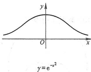
(3) 概率曲线
