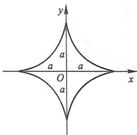
(7) 星形线(内摆线的一种)
